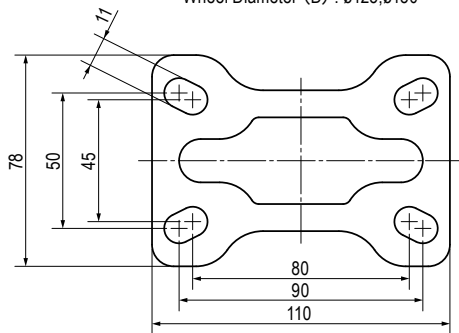
車輪径 (D寸法) が \phi 100 の場合 Wheel Diameter (D) : \phi 100
