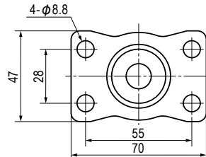
車輪径 (D寸法) が \phi 65 \cdot \phi 75 の場合 Wheel Diameter (D) : \phi 65, \phi 75
