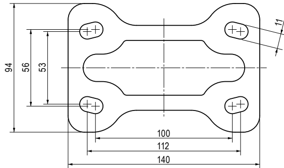
車輪径 (D寸法) が \phi 125 \cdot \phi 150 の場合 Wheel Diameter (D) : \phi 125, \phi 150
