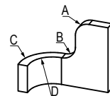
最小曲げ半径説明図 Minmum Bending Radius
