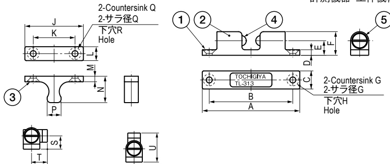
取付例図1
